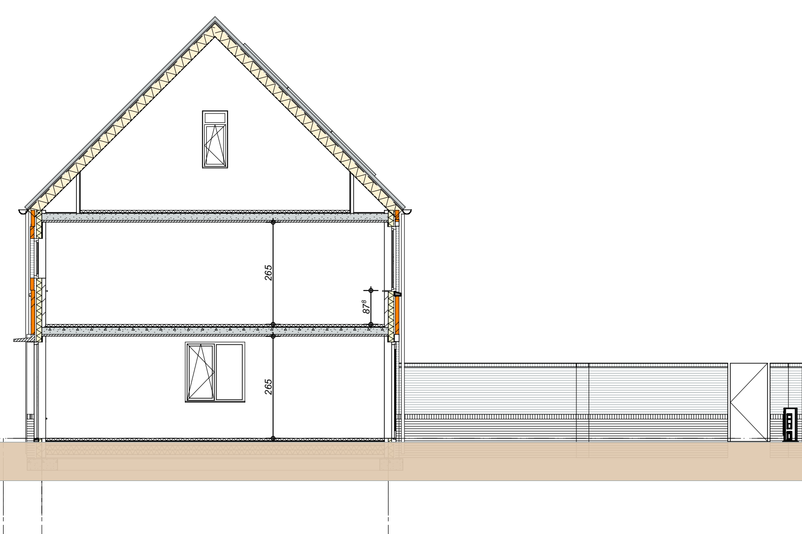
Blok 2 Principe doorsnede A-A 1:100
