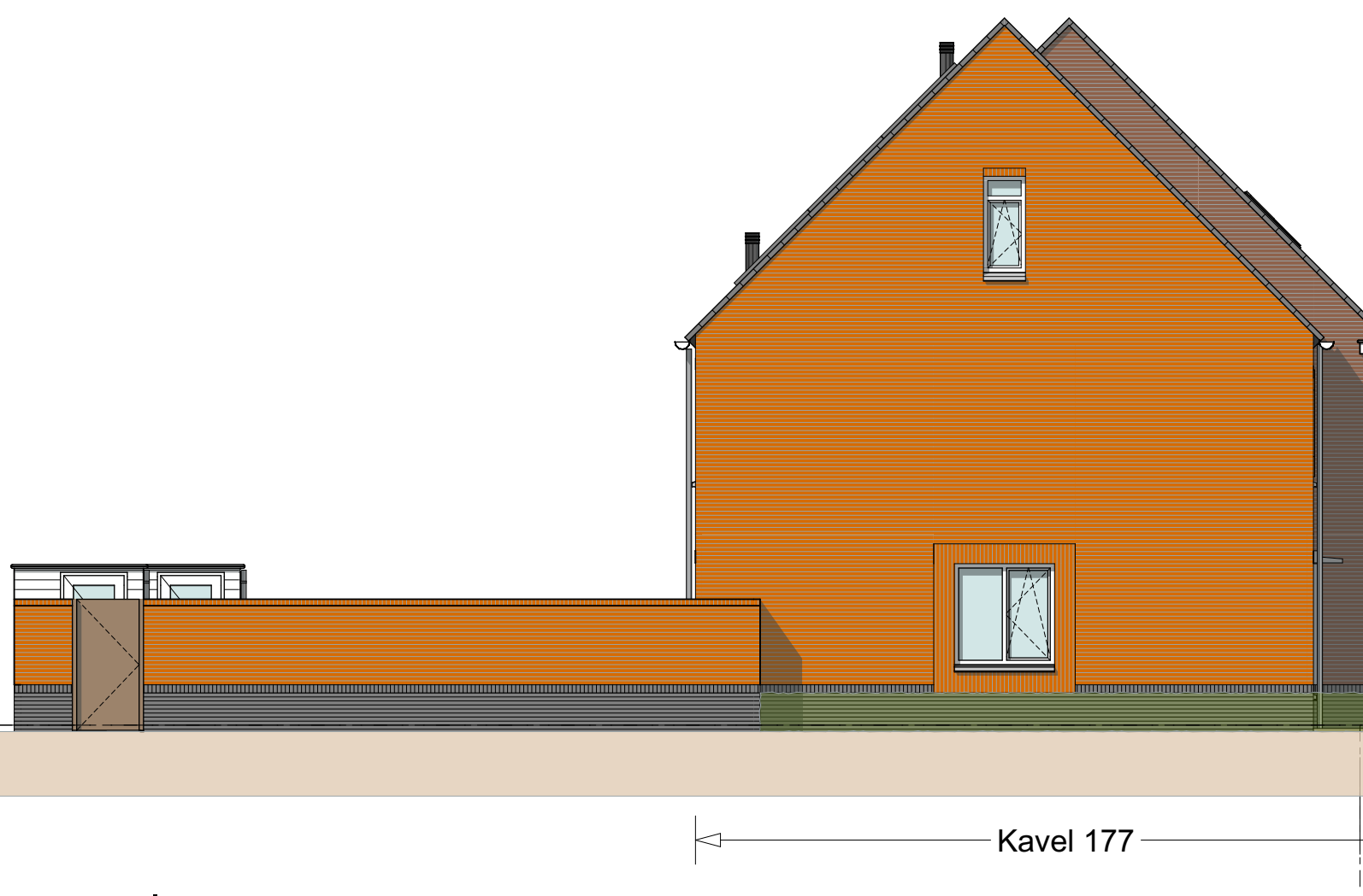
Linkergevel 1:100
