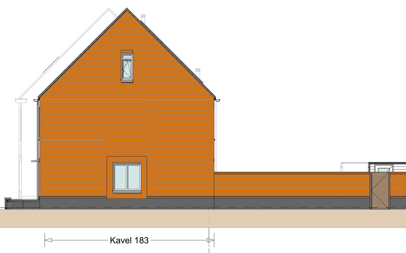
Rechtergevel 1:100
